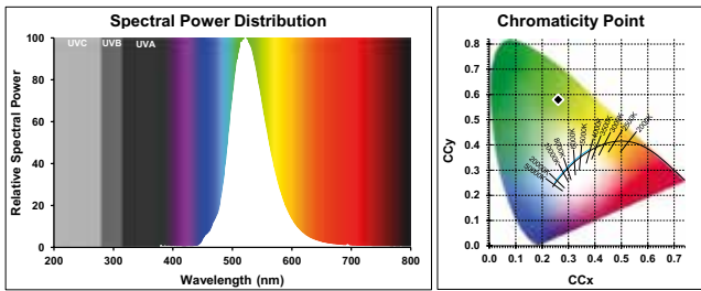
ToLEDo Retro Chroma GLS Green
