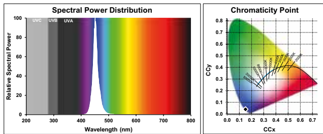
ToLEDo Retro Chroma GLS Blue
